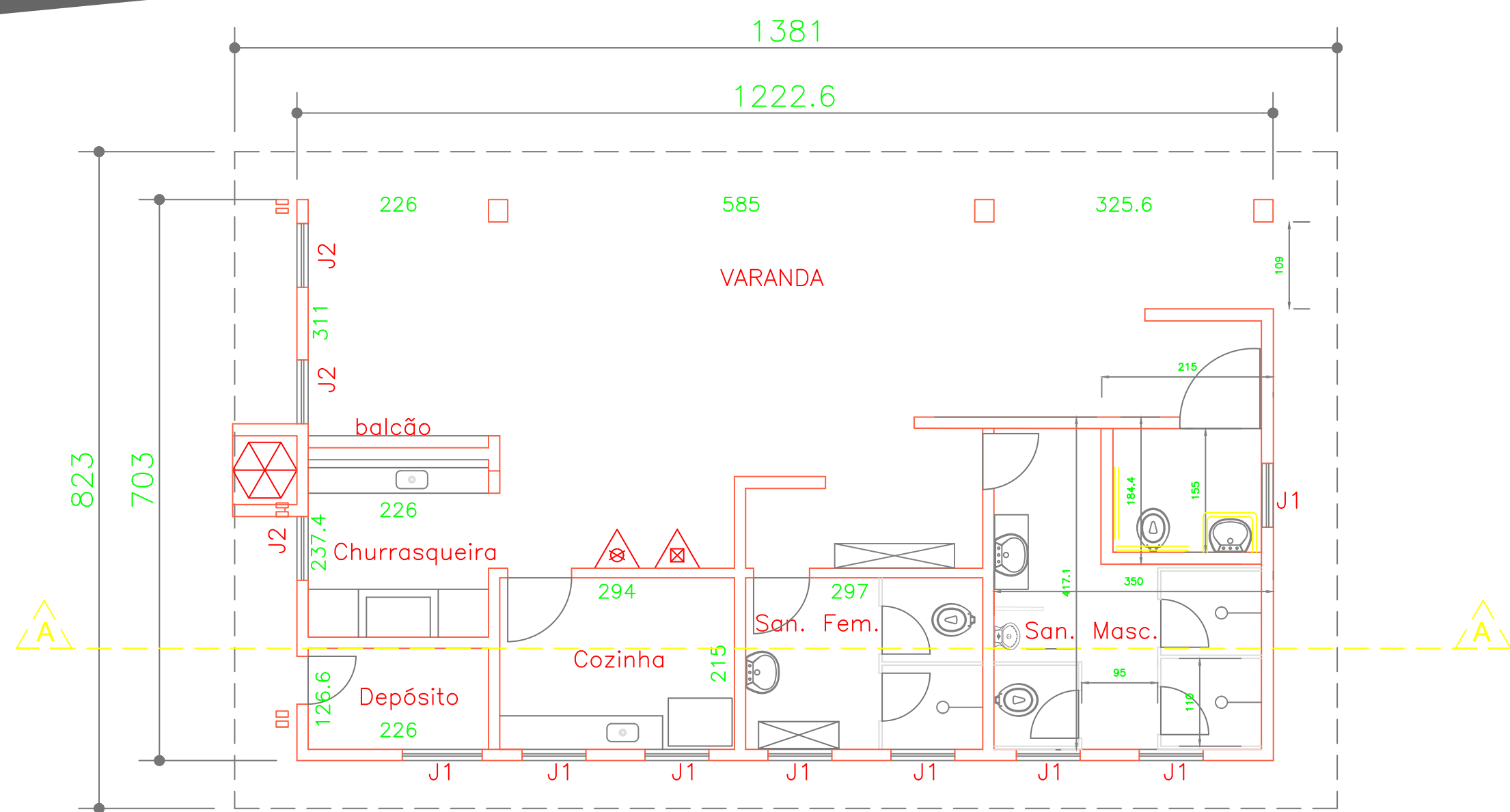
EDIF. 31 - APOIO TAMBORÉU PROPOSTA Planta Baixa ÁREA = 113,65 m² ESCALA 1:200
